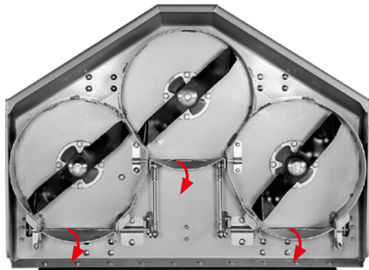
Heckauswurf: offene Schnittkammer Mulch-Modalität: geschlossene Schnittkammer
